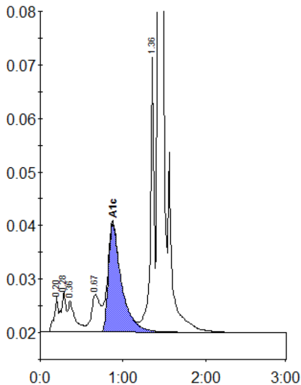
Peak table - ID: 10558157
